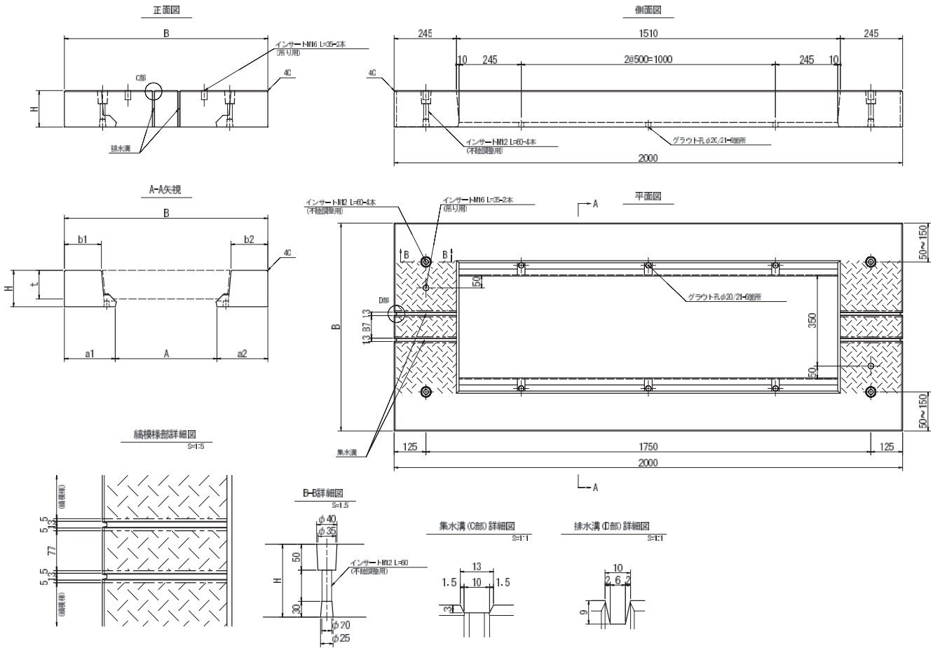
CRスラブⅡ型寸法表
