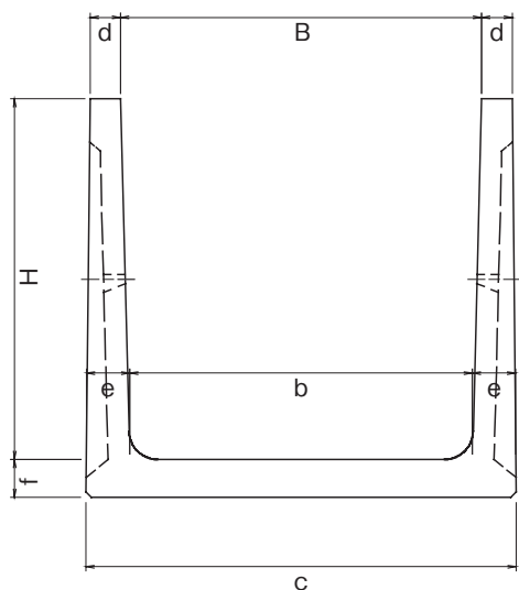
標準型 (N型)
