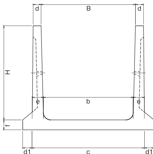
張出型 (NF型)
