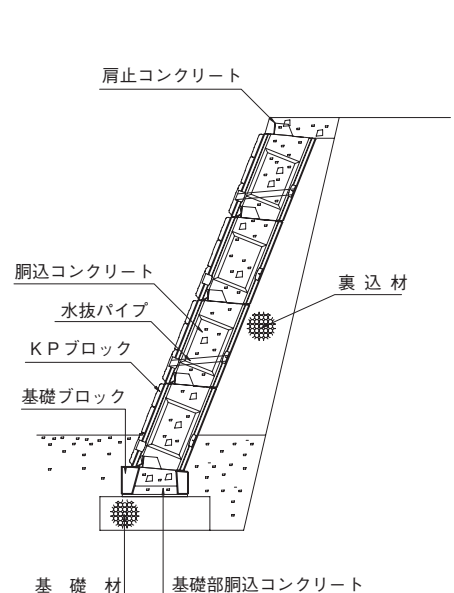
◇断面図
