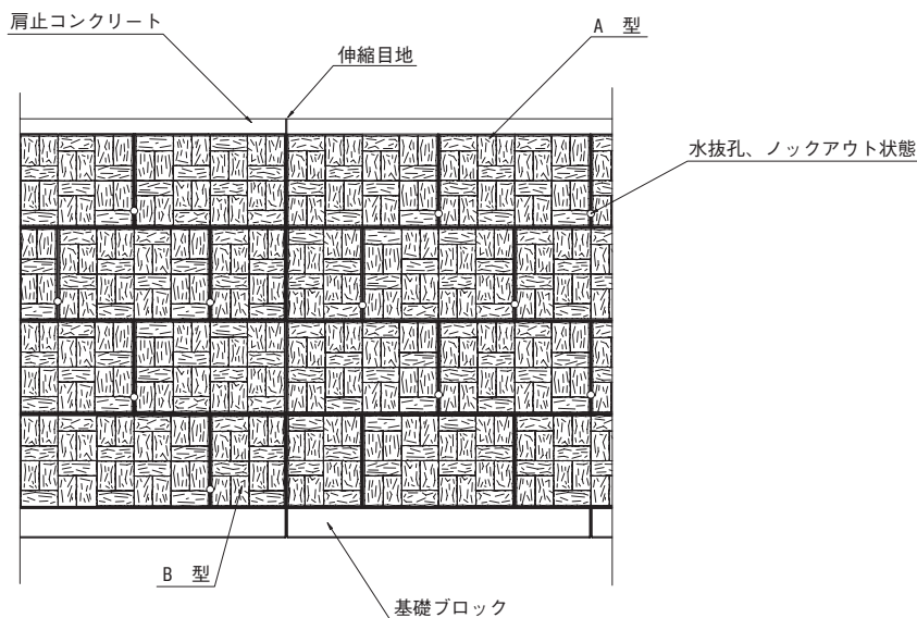
◇正面図
