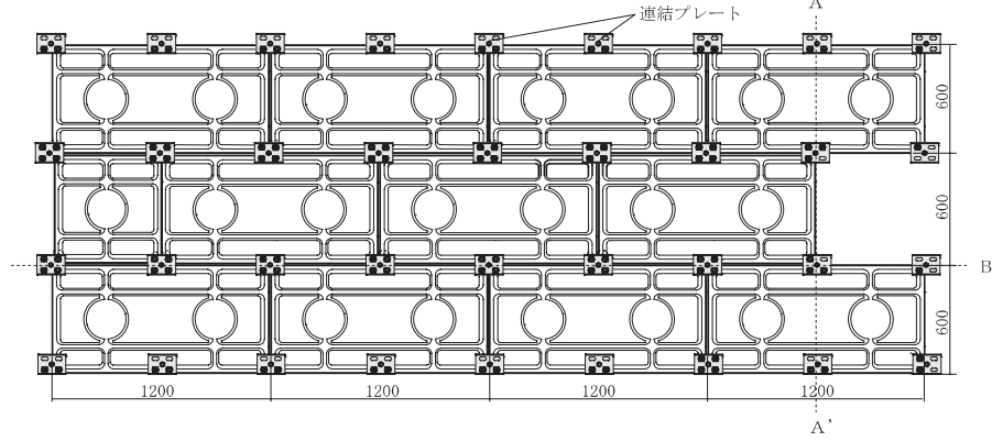
背面図
