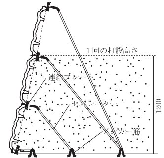
A~A' 断面図
