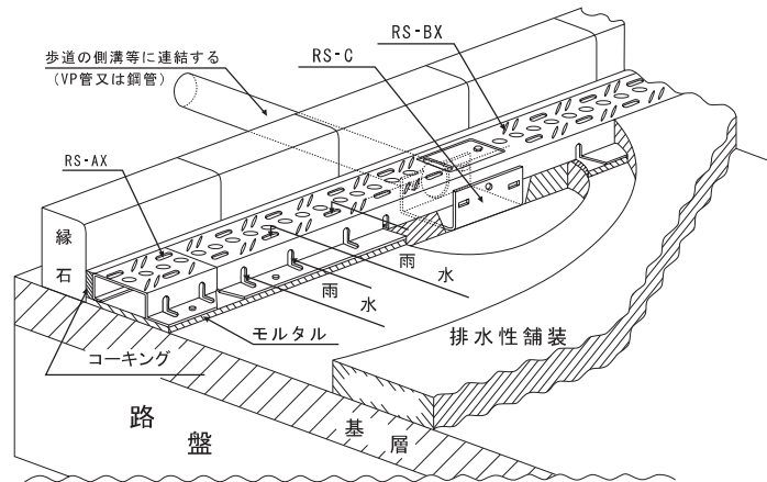
参考標準図
