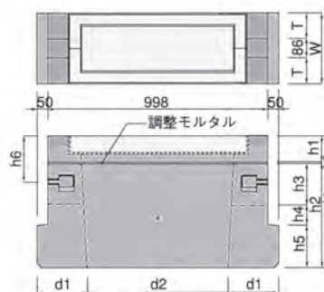
NS-02 φ200~250用
