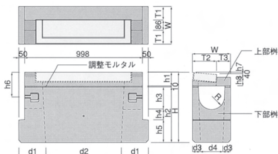
NS-01 φ200~350用
