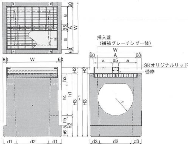
Aタイプ (歩車道ブロック対応)
