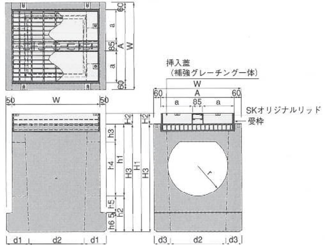
Bタイプ (両面化粧)
