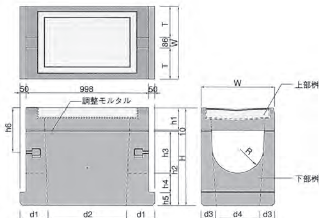
NS-02 φ300~800用
