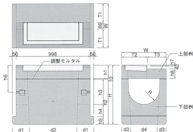
NS-01 φ400~800用
