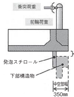
標準設置断面
